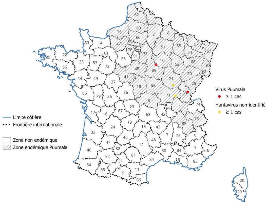
Figure 1 : Distribution spatiale en France métropolitaine des cas confirmés d'infection récente par un hantavirus, diagnostiqués sur la période Janvier 2025 (la distribution des cas se fonde sur la commune du lieu de résidence ou d'exposition si différente ; en hachuré, les départements où des cas d'infection par PUUV ont été détectés sur la période 2012-2024; la superposition de cas privilégie les cas où l'hantavirus a été identifié).
